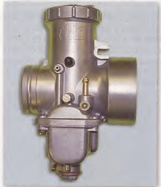
Carburador de tiro horizontal
